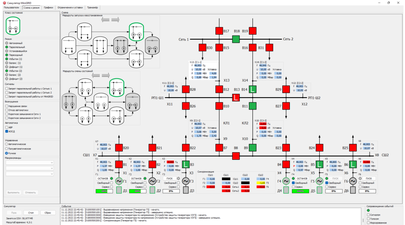
Рисунок 8.2.2.1 – Видеокадр «Схема и режим»
