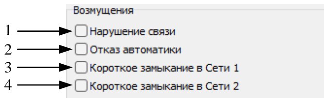
Рисунок 8.2.2.5 – Видеокадр «Схема и режим». Панель «Возмущения»: 1 – метка нарушения связи с Сетью; 2 – метка отказа автоматики МиниGRID; 3 – метка короткого замыкания в Сети 1; 4 – метка короткого замыкания в Сети 2
