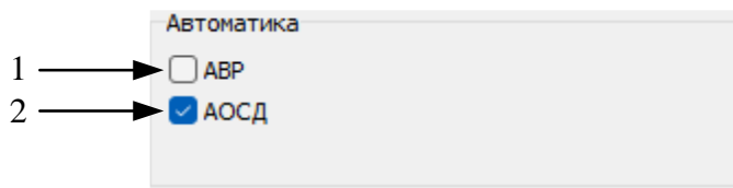
Рисунок 8.2.2.6 – Видеокадр «Схема и режим». Панель «Автоматика»: 1 – метка включения/выключения автоматики ввода резерва (АВР) от внешней сети; 2 – метка включения/выключения автоматики опережающего сбалансированного деления (АОСД)
