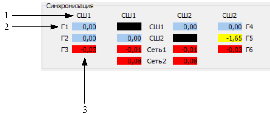
Рисунок 8.2.2.11 – Видеокадр «Схема и режим». Панель «Синхронизация»: 1 – наименование «первого» источника; 2 – наименование «второго» источника; 3 – разница фаз напряжения между источниками
