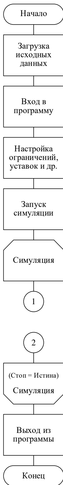
Рисунок 4.1.1 – Алгоритм программы
