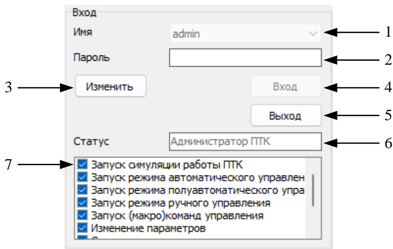
Рисунок 8.2.1.3 – Видеокادر «Пользователи». Панель «Вход»: 1 – разворачивающийся список имён зарегистрированных пользователей; 2 – поле ввода пароля пользователя; 3 – кнопка изменения пароля; 4 – кнопка входа пользователя; 5 – кнопка выхода пользователя; 6 – статус пользователя; 7 – права пользователя
