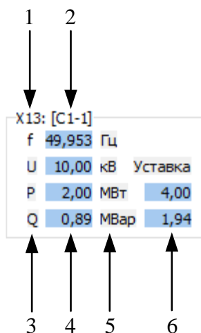
Рисунок 8.2.2.14 – Видеокадр «Схема и режим». Панель «Точка контроля в сечении»: 1 – наименование точки контроля; 2 – наименование сечения; 3 – обозначения контролируемых параметров; 4 – значения контролируемых параметров; 5 – единицы измерений контролируемых параметров и уставок; 6 – значения уставок
